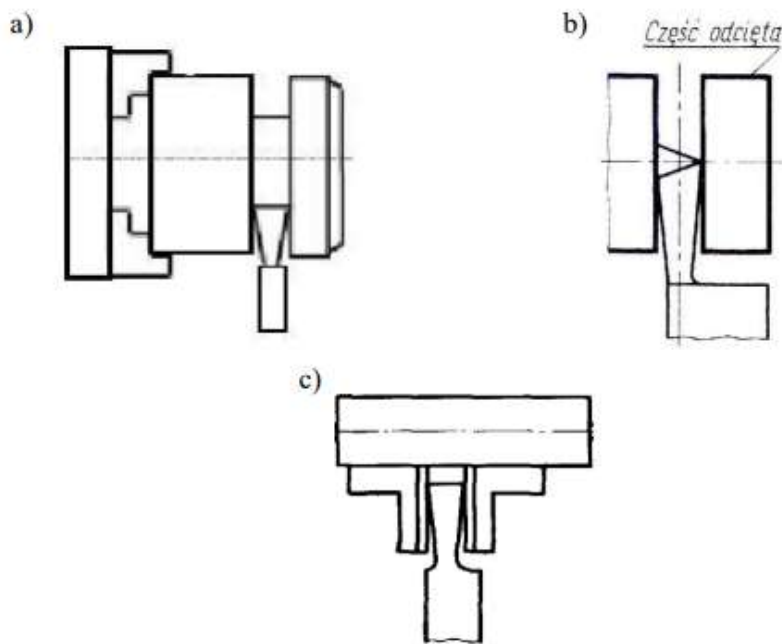
Toczenie poprzeczne: a) nacinanie rowka, b) przecinanie, c) ustawienie noża przecinaka [2].
